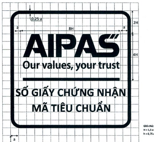
Hình 03: Kích thước mẫu dấu Chứng nhận hợp chuẩn.
